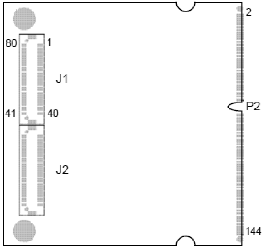
Bottom Side
